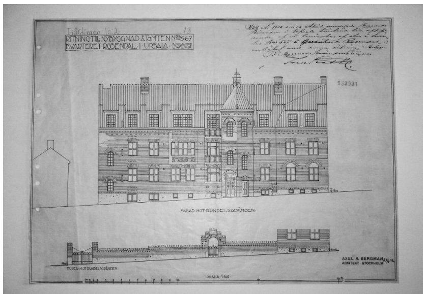
Fasadritning (notera skillnaderna, bl.a. i muren mot den uppförda)
