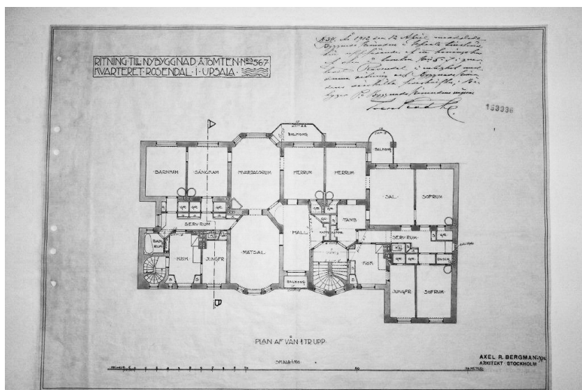
Planritning av våning 1 trappa (notera att paradvåningen har burspråk även i matsalen).
