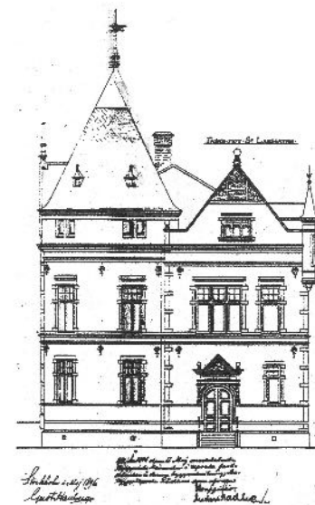
Gerdt Hallbergs förslag från 1896 som inlämnades till Uppsalas byggnadsnämnd för godkännande.
